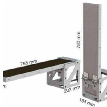
Nedfellbart Skrustikkestativ
