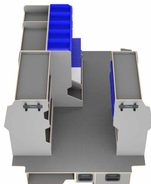
Elektrikerinnredning sett ovenfra
