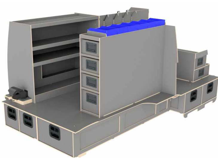
Innredning sett bakfra
