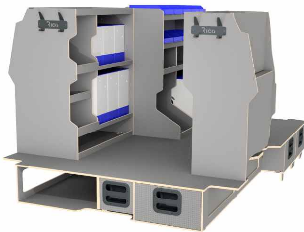
Elektrikerinnredning med plass til gardintrapp i gulv
